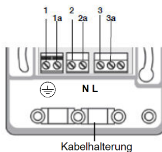
Abbildung 4: AC-Schalter (mit Zähler) Anschlüsse
