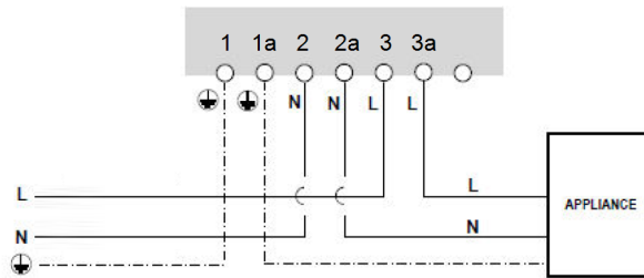
Abbildung 5: Anschluss an das Gerät
