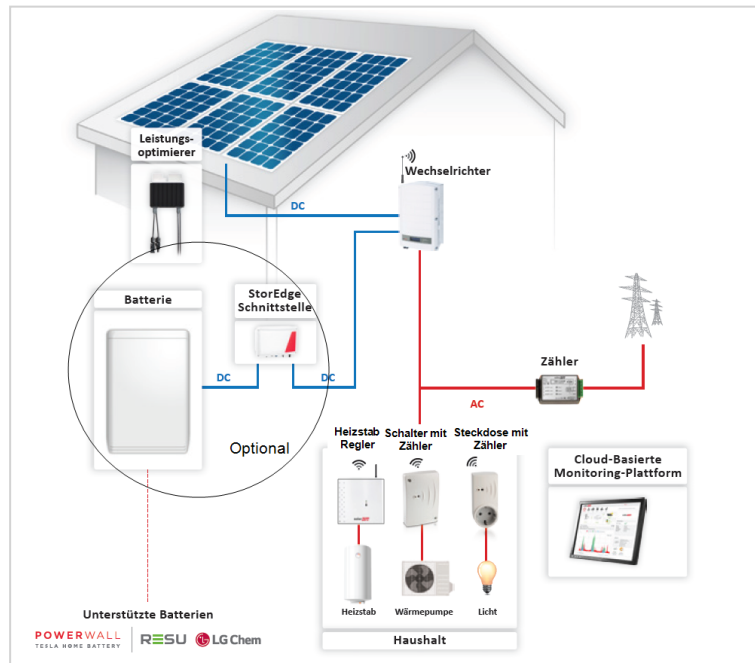
Abbildung 1: SolarEdge-System mit Hausautomation
